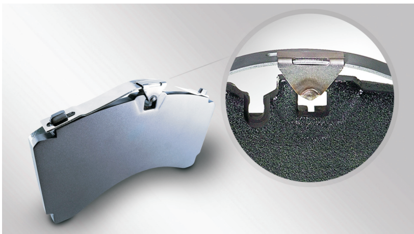
ProTecS® systém zajištění brzdových desek: brzdové desky s navařeným držákem.
