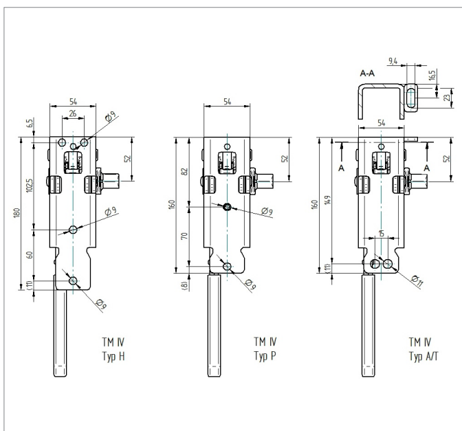
HESTAL TensionMaster IV výkres variant montážních otvorů
